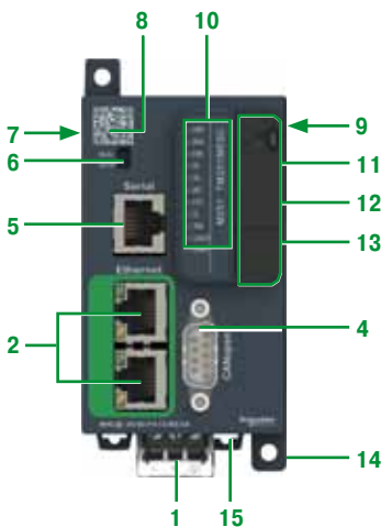
Контроллер TM251MESB
